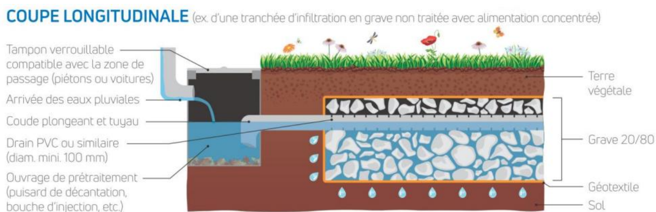
Figure 65. Coupe longitudinale de la tranchée d'infiltration
