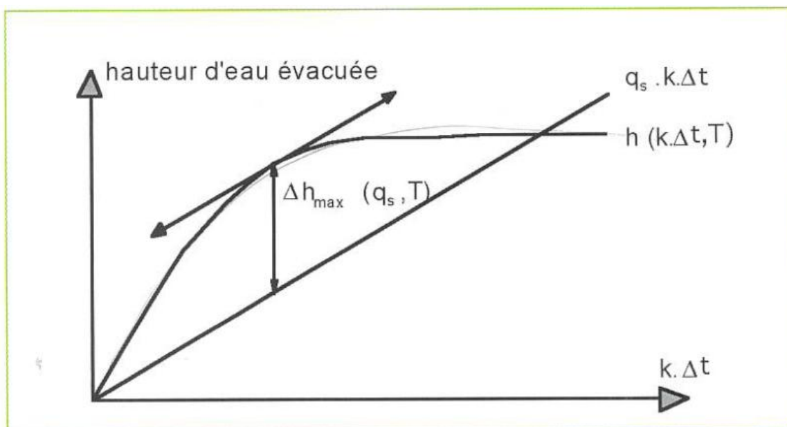
Figure 61. Superposition de la courbe Hauteur-durée pour une fréquence choisie et la courbe d'évacuation
